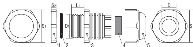
Фиксирующая гайка 1, уплотнитель 2, корпус 3, прокладка 4, гайка уплотнения 5.
