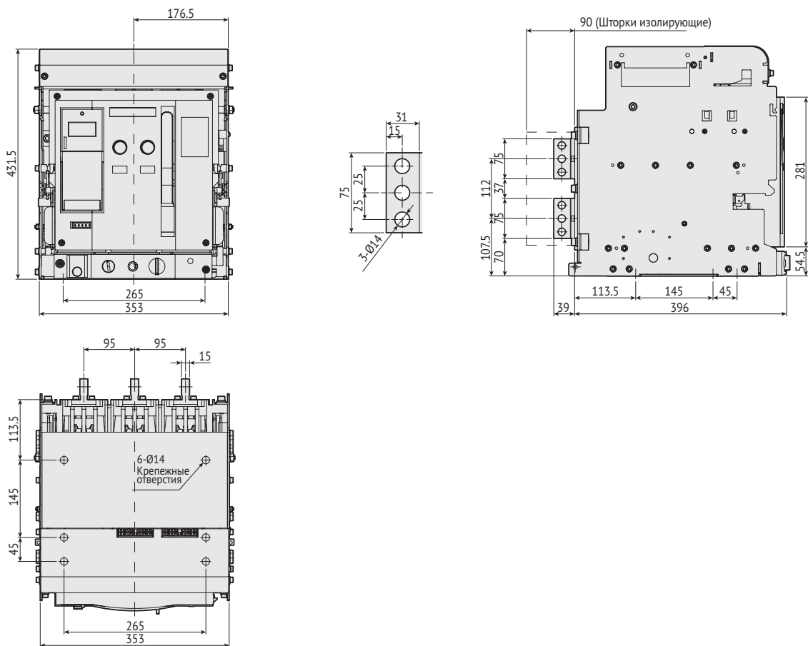
Рисунок А.6 - Автоматический выключатель OptiMat-S2 выдвижного исполнения на номинальный ток 2000 А заднего присоединения.
