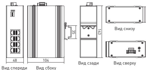
Рис. 1 — Габаритные размеры TSX-U-8GT
