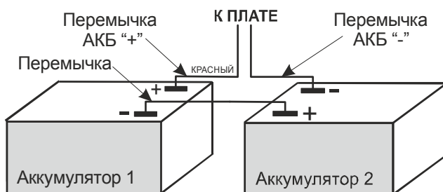
Рисунок 5 – подключение АКБ
